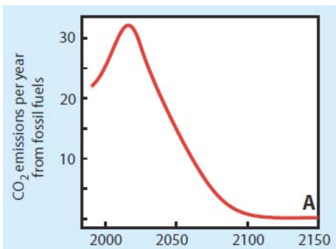
Рис.1 А: Уровень выбросов \text{CO}_2 от использования ископаемых видов топлива по сценарию предотвращения изменений климата, предполагающему к 2050 г. сокращение уровня выбросов ПГ (включенных в Киотский протокол) на половину относительно уровня 2000 г. (Schellnhuber, 2008) 17
